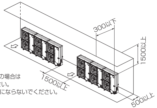
(5) 1台多列設置の場合
