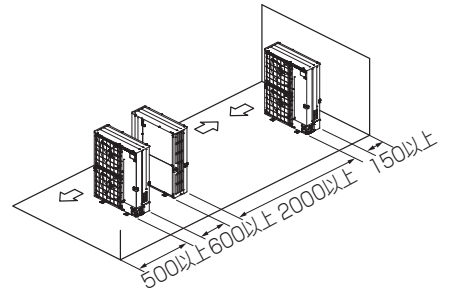
(5) 1台多列設置の場合
