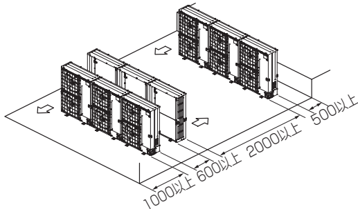
(6) 複数台多列設置の場合
