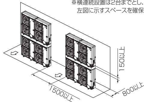
(7) 段積み設置の場合
