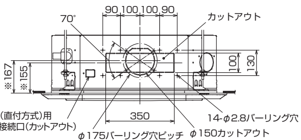
分ダクト接続口断面図
