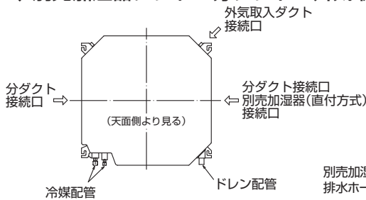
外気取入口詳細図
