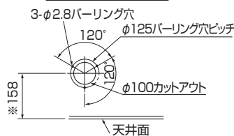
外気取入口詳細図
