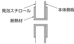
分ダクト接続口断面図
