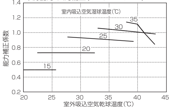
冷房能力・入力補正(オールフレッシュ)
