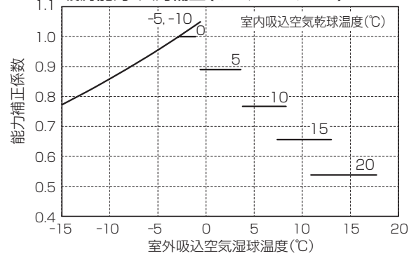
暖房能力・入力補正(オールフレッシュ)
