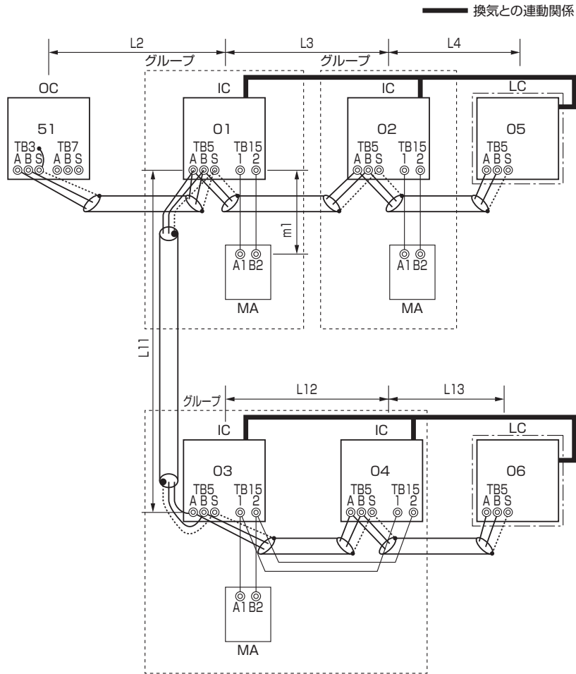
制御線配線例
