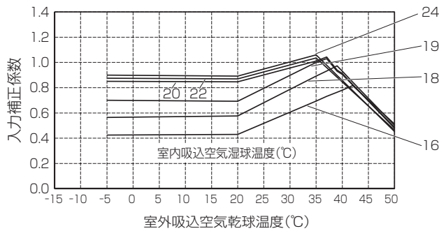
冷房能力・入力補正(オールフレッシュ)
