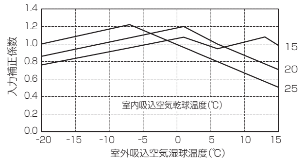
暖房能力・入力補正(オールフレッシュ)
