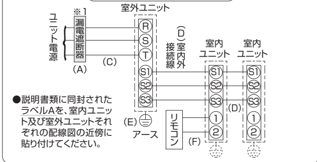
同時ツインシステムの配線
