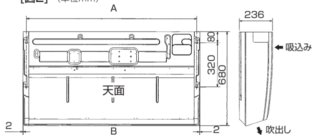
[図2] (単位mm)
