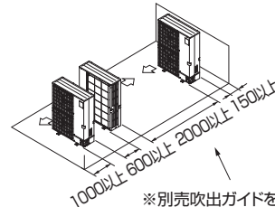
(5) 1台多列設置の場合
