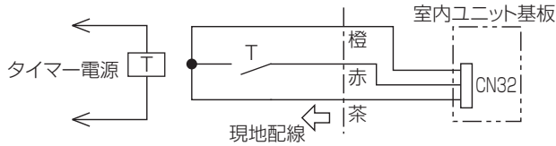
【基本配線図】
