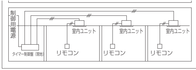
【基本配線図】
