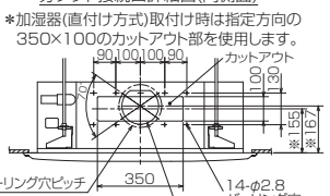
分ダクト接続口詳細図(両側面)
