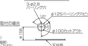
カンタン自動パネルの場合 別売ワイヤレス受光部キット取付の場合(社名表示部)
