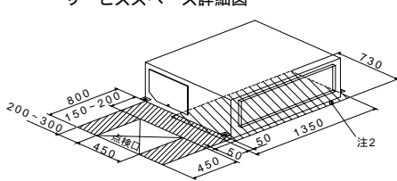
サービススペース詳細図
