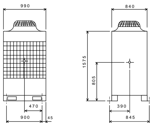
PUHY-P500 · P560 · P630 · P670 · P730SM-E形
