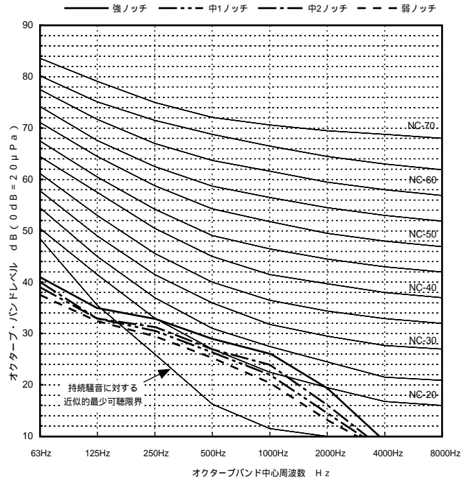
PLFY-P71AM-E1形
