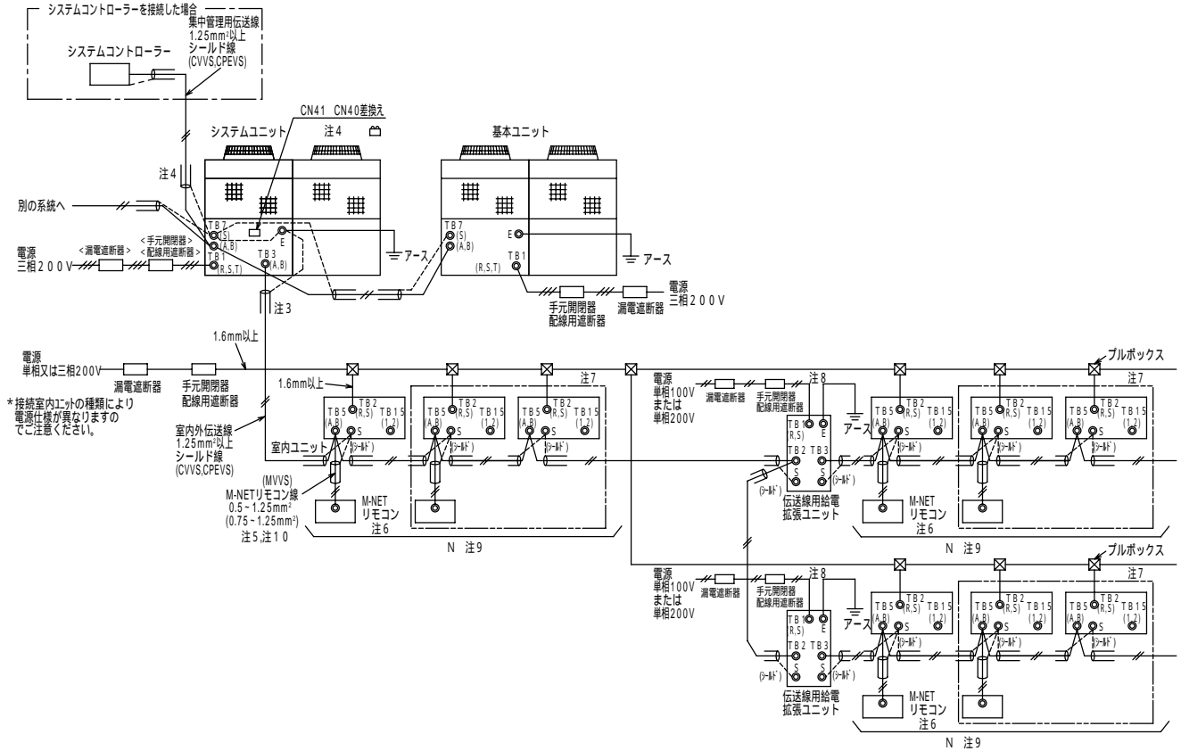
M-NETリモコンを用いたシステム
