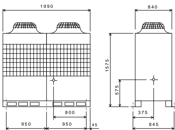
PUHY-P450 · P730KM-E形
