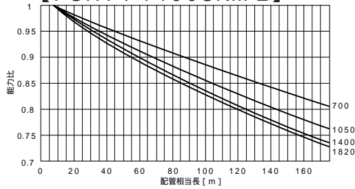
【PUHY-P1400SKM-E】
