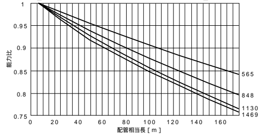
【PUHY-P1240SKM-E】
