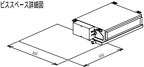
サービススペース詳細図
