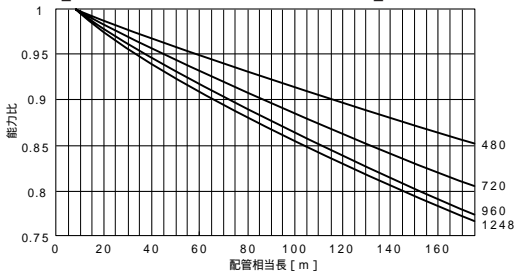
【PUHY-P1080SKM-E】
