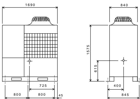
PVHN-P100SM-E形
