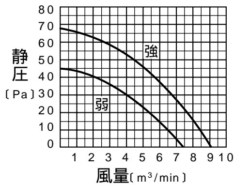
2方向吹出し（ベーン水平）角形ダクト
