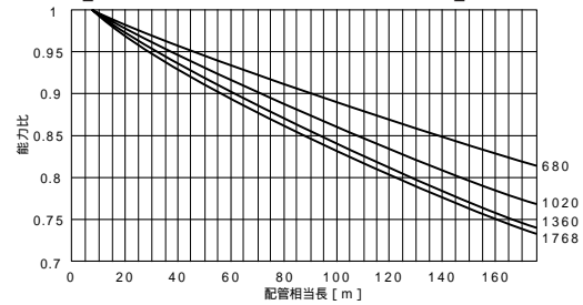
【PUHY-P1360SKM-E】
