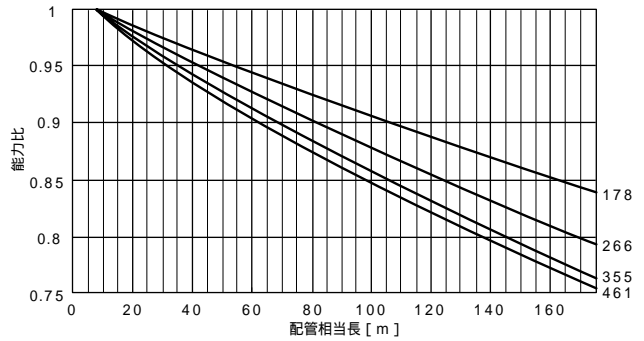
【PUHY-P355M-E】
