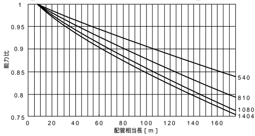
【PUHY-P1180SKM-E】
