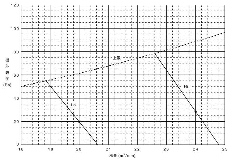
PLFY-P71・80CLMD-E1
