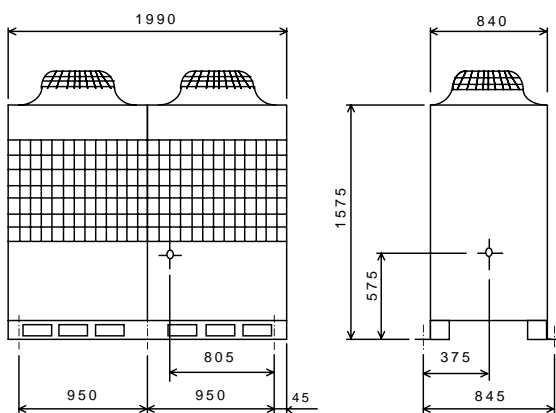
PUHY-P450 · P730KM-E形
