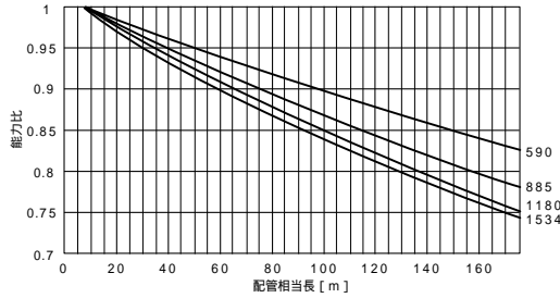
【PUHY-P1300SKM-E】
