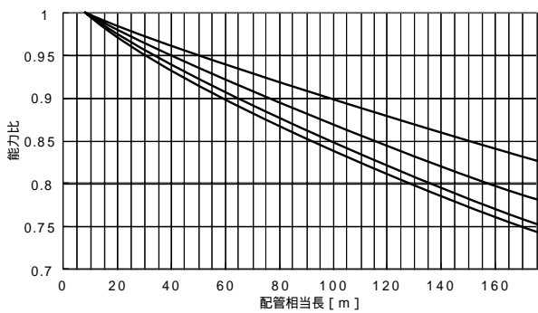
【PUHY-P400M-E】
