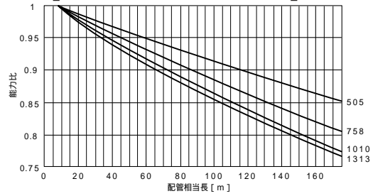
【PUHY-P1130SKM-E】
