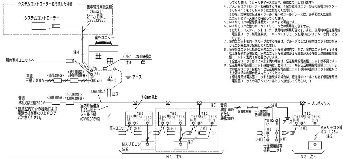
MAリモコンを用いたシステム
