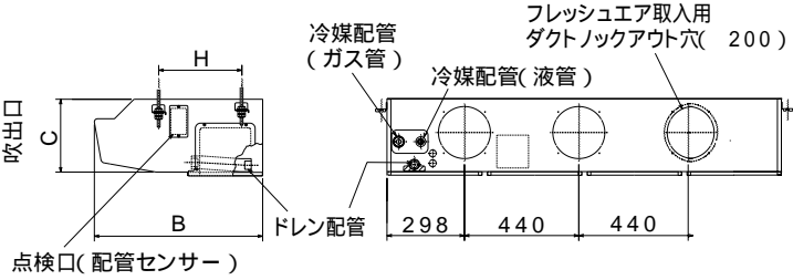
P80形の場合
