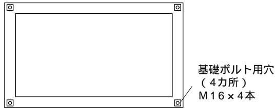
図1 PFAV-P1120・P1400・P1600形基礎図
