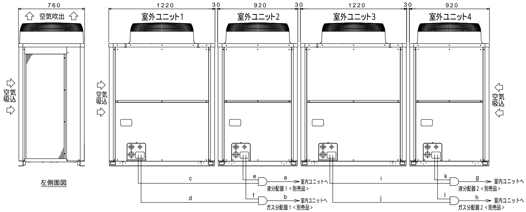
正面図
