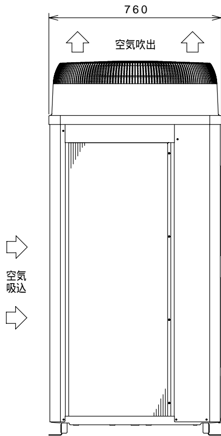
左側面図
