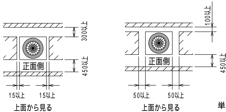
後面側、壁面まで300mm以上の場合
