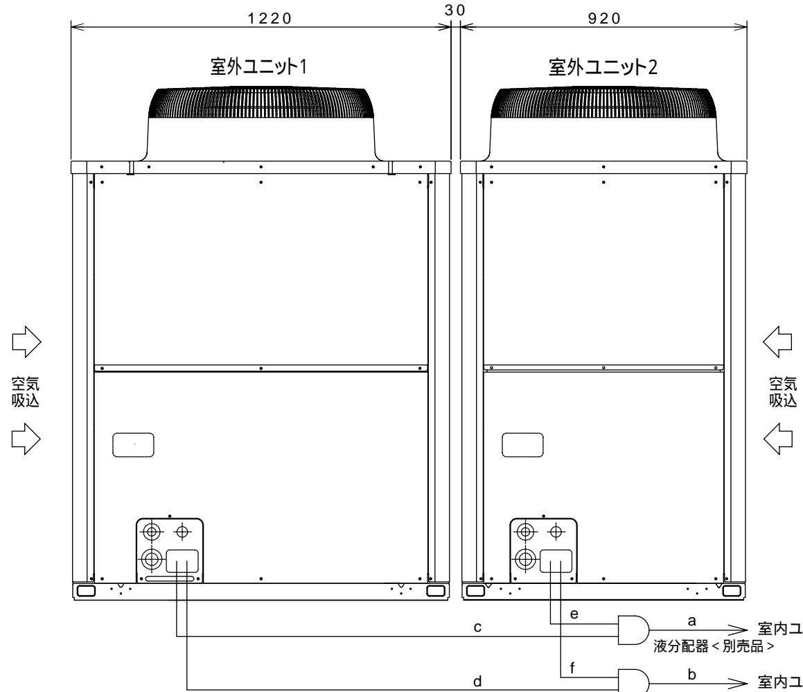
正面図
