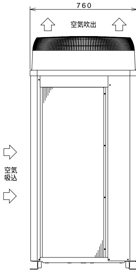
左側面図
