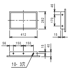
外気取入フランジ 別売部品
