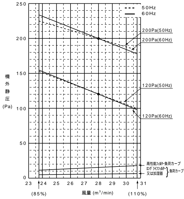
PEFY-P224M-E1-F
