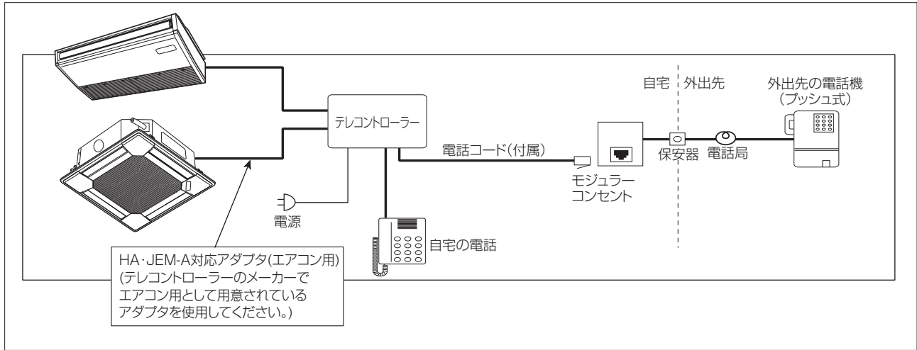
[テレコントロールシステム系統図]
