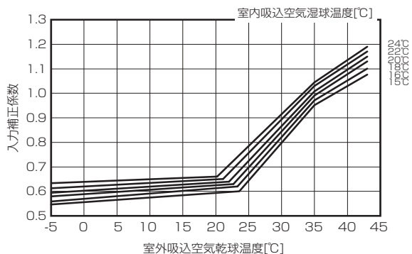
③冷房温度補正 (室温サーモ形給気処理ユニット、外気処理エアコン)
