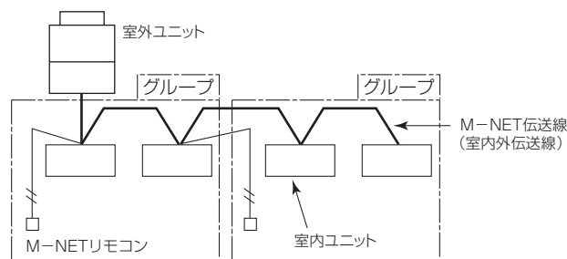
< M-NET リモコンを使用した場合 >
