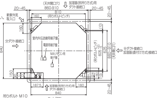
加湿器(別吊り方式)用ダクト接続口詳細図(両側面)
