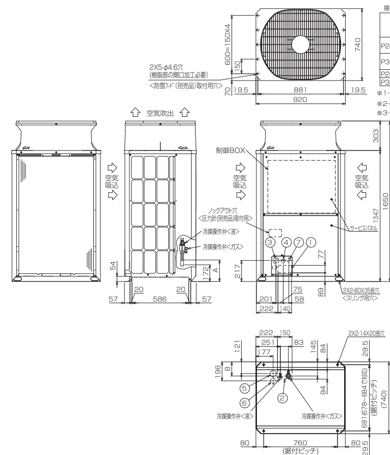
接続管仕様
