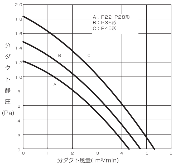
■PLFY-P22・P28・P36・P45LMG1
