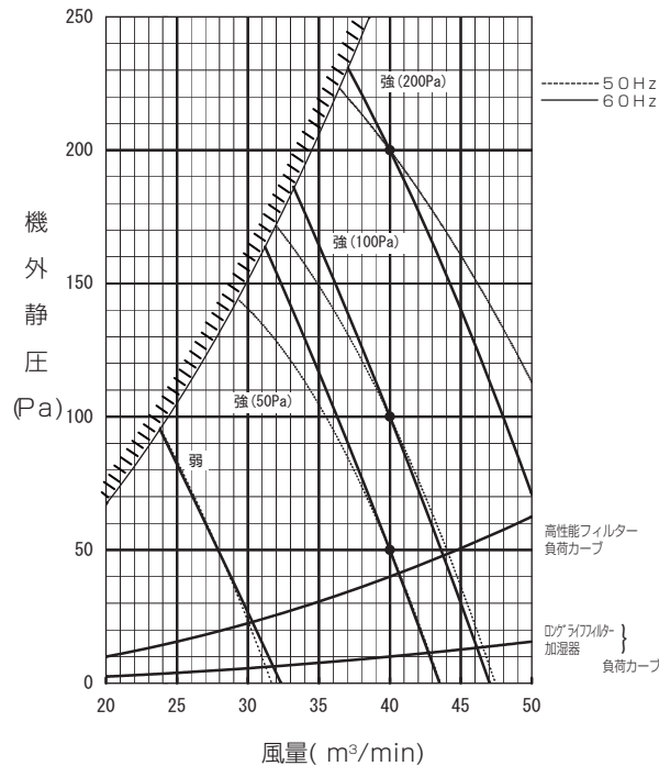
■PEFY-P160MG2
