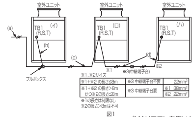
(MAリモコンを用いたシステム)
