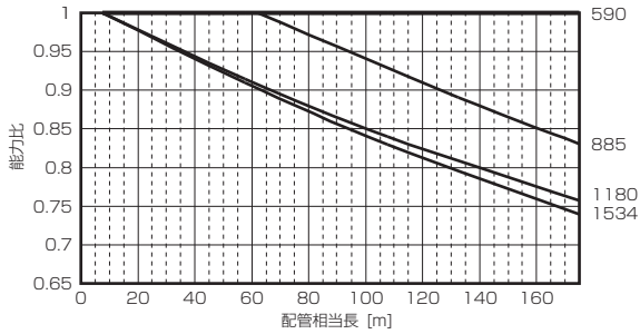
■PUHY-EP1300SDMG2
