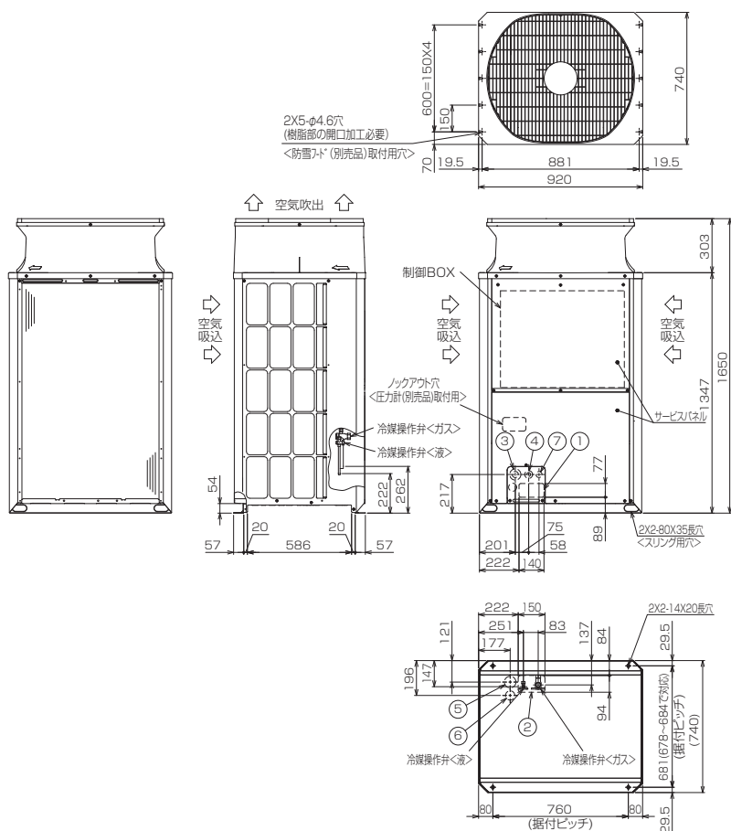
接続管仕様
