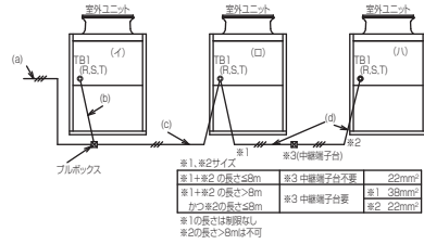
図1 (MAリモコンを用いたシステム)
