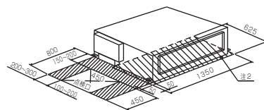
サービススペース詳細図
