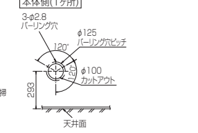
新鮮外気取入口詳細図
