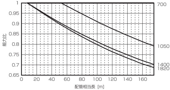
■PUHY-EP1400SDMG2
