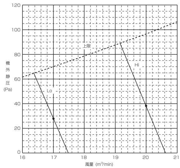
■PLFY-P45・56CLMG1
