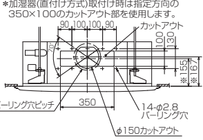
分ダクト接続口詳細図(両側面)
