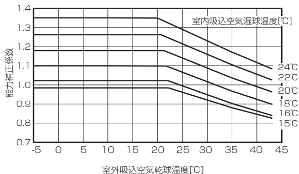
①冷房温度補正
