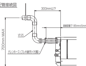
ドレン配管接続図
