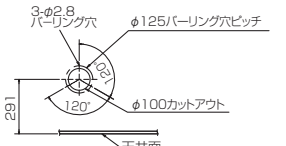
分ダクト接続口詳細図(両側面)
