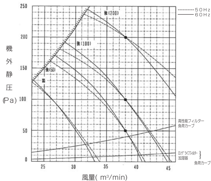
■PEFY-P112・140MG2
