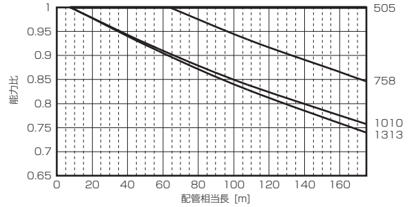
■PUHY-EP1130SDMG2
