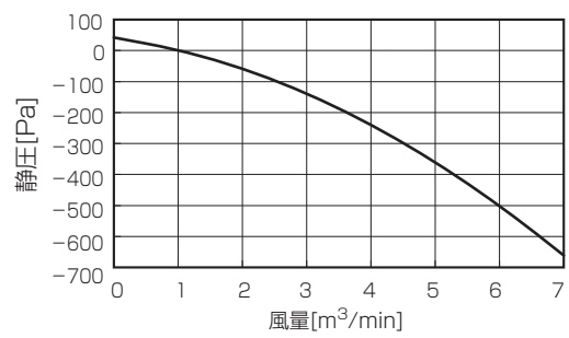
フィルターケースメント+高性能フィルター
