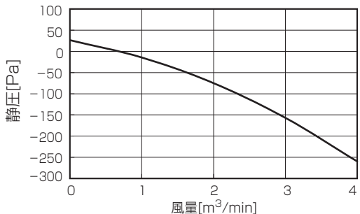
標準フィルター
