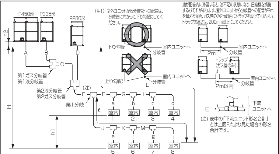
接続例 (室内ユニットを8台接続の場合)
