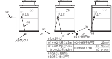
(MAリモコンを用いたシステム)
