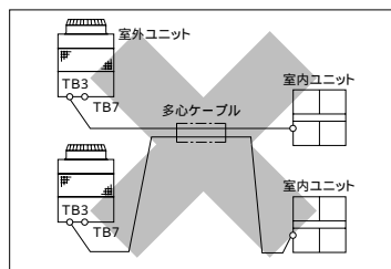
TB3:室内外伝送線用端子台、TB7:集中管理用伝送端子台
