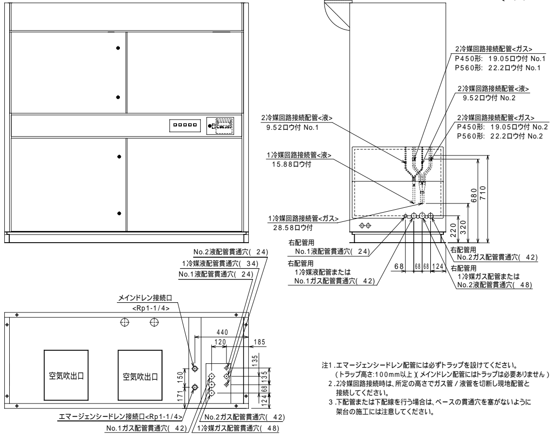
床面寸法図
