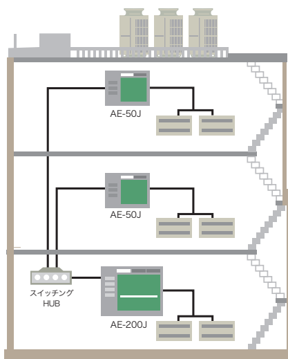
「AE-200J」1台と「AE-50J」2台を併用して、81台の室内ユニットを制御
