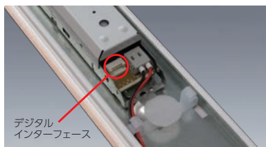
ライトユニット裏側
