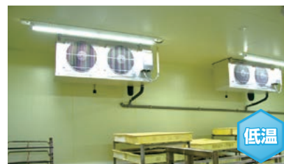
餡冷却室に設置されたユニットクーラで、製品の粗熱を除去
