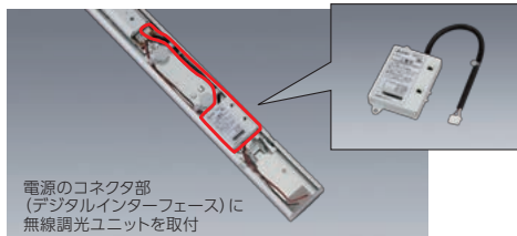
電源のコネクタ部(デジタルインターフェース)に無線調光ユニットを取付 ※前タイプの110形ライトユニットには無線調光ユニットが2つ必要です。
