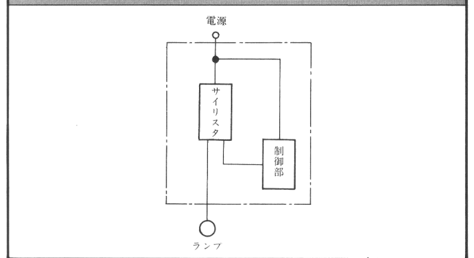
ダイヤフラッシャーの系統図
