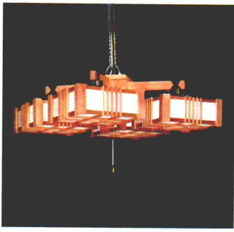
ルミホーム610B (ルミクリスタル) 10畳 ◎ ¥53,200 M37S25 30W形円形蛍光灯×4 ●吊具C-44 ¥11,200 ①M7S85 ●灯具FCP3201×4 ¥10,500×4 ④M7S35×4 木製枠 和紙入りプラスチックセード プルスイッチ・豆球つき 外径φ880 吊り高さ246~676 重さ8.1kg
