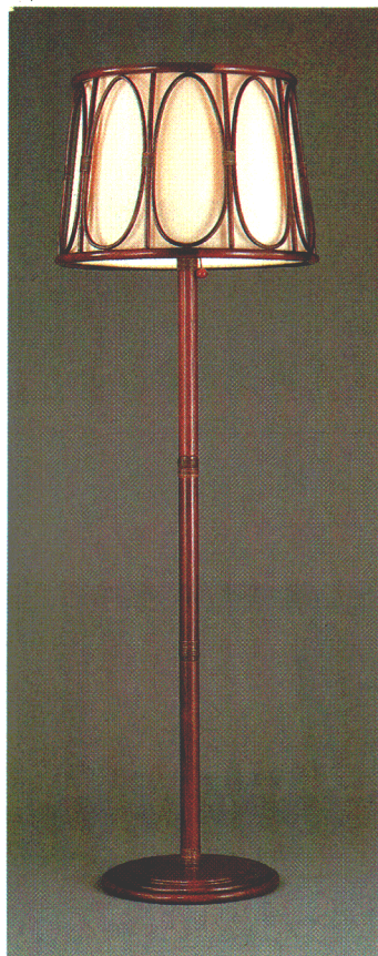
ルミチャーム614 ㉔ ○¥65,000 M46S8 100W形電球 (E26) (本体 H6014 ○¥31,400 ①M22S6) (セード F1014 ○¥33,600 ①M24S2) 藤製枠 布セード プルススイッチ・豆球つき セード幅φ500 セード高さ350 高さ1510
