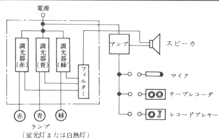
カラーミュージックライトの系統図
