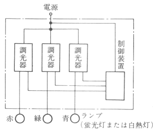
オートカラーチェンジャー系統図
