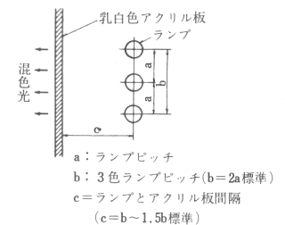
オートカラーチェンジャーの照明手法例
