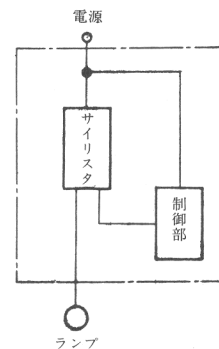
ダイヤフラッシャーの系統図
