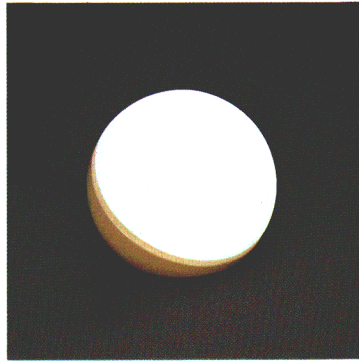
LB421Y ○¥8,500 ①M6S1 25W電球 (ミニランプ) (E17) 乳白ガラスグローブ 黄色陶器本体 スイッチつき 幅φ144 高さ125
