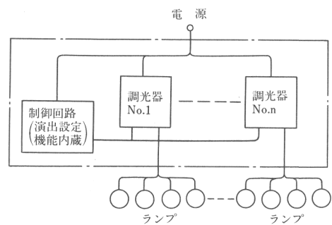
ダイヤフラッシャーの系統図
