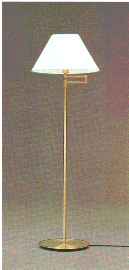
ルミチャーム625 ㊸ ○¥56,000 100W形電球(E26) ●本体 H6025 ¥38,000① ●セード F1025 ¥18,000① 白色布セード 金色メッキ本体 水平可動アーム プルスイッチつき 幅φ450 高さ1400
