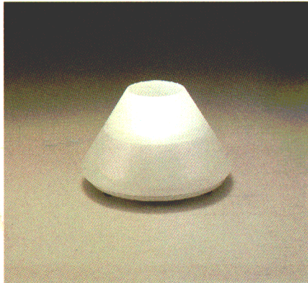
LB456S (NEW) ○¥18,200 ① 50Wハロゲンランプ(12V)(GY6.35) すりガラスセード クロム色塗装本体 スイッチつき 幅φ200 高さ130 ●電子ダウントランスつき
