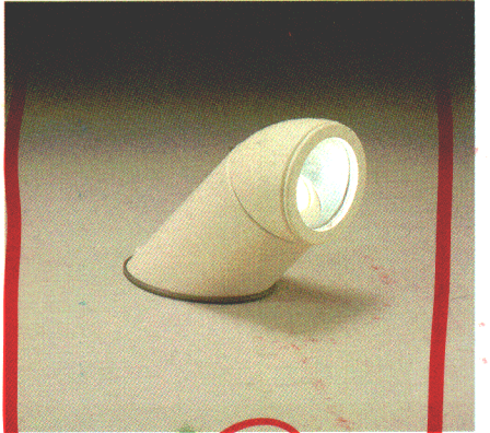
LB458 (NEW) ○¥28,600 ① 20Wハロゲンランプ(12V)(G4) 白色メタルセード 白色メタル本体 アルミ反射板銀色梨地仕上げ スイッチつき 幅φ153 高さ128 ●電子ダウントランスつき
