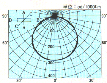
配光曲線
