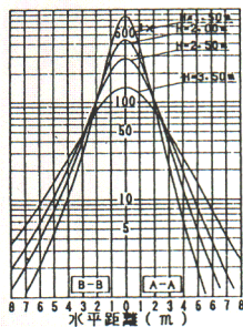
水平照度
