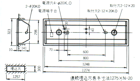
連続埋込穴長手寸法1275×N-20 (Nは器具台数を示します。)
