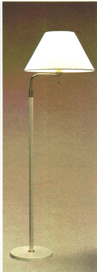
ルミチャーム622W (B) ○¥42,500 100W形電球 (E26) ●本体 H6022W ¥27,500① ●セード F1022W ¥15,000① 白色布セード 白色塗装本体 プルスイッチつき 幅φ450 高さ1420
