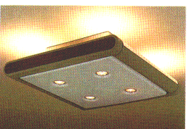
ダイクロックミラー付きハロゲンランプ60W×4ミニランプ40W×4
