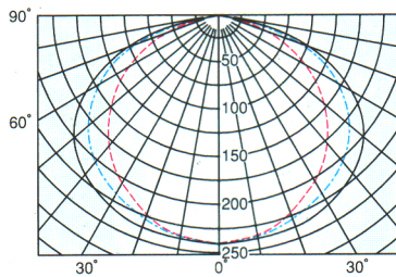
配光曲線 (SY4032) (cd/1000ℓm)
