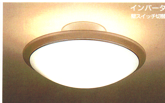
ZML7 ¥57,800 ① ●(32W+40W)形円形ルピカ蛍光灯(エース色)+40W形円形ルピカ蛍光灯(電球色) ●乳白アクリルカバー(帯電防止仕様) ●ダークベージュメタリック塗装仕上 ●壁スイッチ切替(全光・直接光・間接光・常夜灯・消灯) ●外径φ600 全高250 重4.0kg
