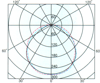
配光曲線 (cd/1000ℓm)
