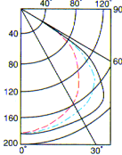
配光曲線
