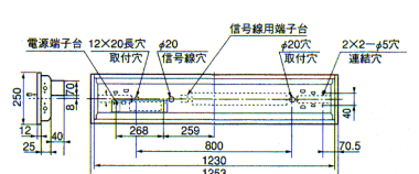
埋込穴 220 × 1235 ★連続埋込穴長手寸法 1253 × N-18 (Nは器具台数を示します)
