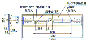
埋込穴 220 × 1235 ★連続埋込穴長手寸法 1253 × N-18 (Nは器具台数を示します)
