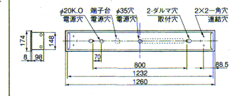
埋込穴 150×1235 ★連続埋込穴長手寸法 1260×N20 (Nは器具台数を示します)
