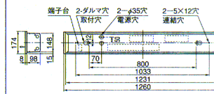
埋込穴 150×1235 ★連続埋込穴長手寸法 1260×N20 (Nは器具台数を示します)
