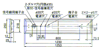
下面開放形 蓄電池内蔵形
