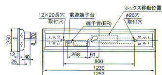
下面開放形 電源別形
