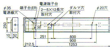
下面開放形
