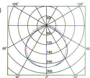
配光曲線 (cd/1000lm)
