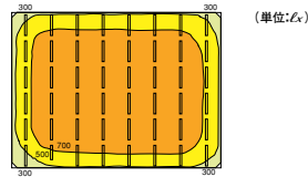
マルチファインルーバ L4221A取付時
