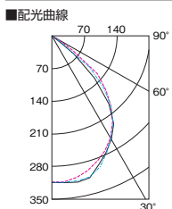
YB2062F+L2842Aの場合 配光 横方向 30度 縦方向 30度
