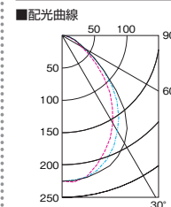
YB2062F+L2862Aの場合 配光 横方向 30度 縦方向 30度
