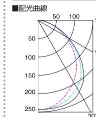
YB2062F+L2872Fの場合 配光 横方向 15度 縦方向 15度
