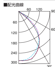
YB2062F+L2852Aの場合 配光 横方向 30度 縦方向 30度
