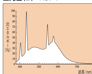
昼光色(D) Ra74
