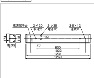
確認図番(EF08029)
