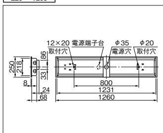
確認図番(EF08034)
