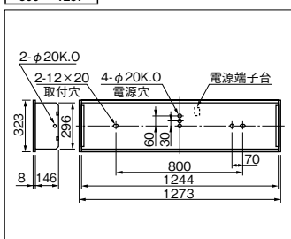
確認図番(EF08033)
