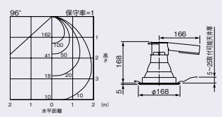
直射水平面照度 使用ランプ：FDL13EX-N
