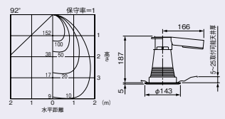
直射水平面照度 使用ランプ：FDL18EX-N
