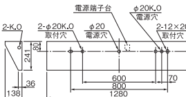
直付形 FHF 32W x 3
