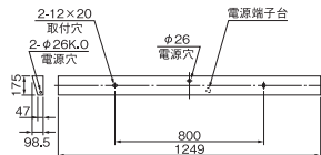
直付形 FHF 86W x 2
