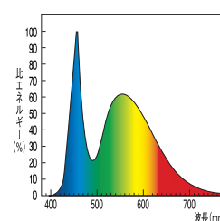
LDA5D-H-E17(昼光色)
