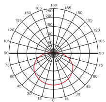
LDA12L-H/D(電球色)
