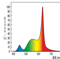
LDA12L-H/D(電球色)
