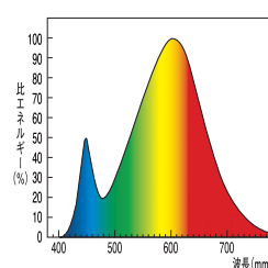
LDA5L-H-E17(電球色)
