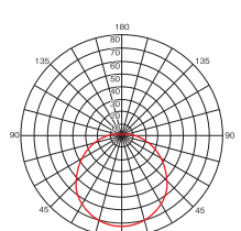
LDA5L-H-E17(電球色)
