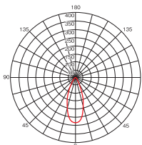
LDR5L-W-E17(電球色)
