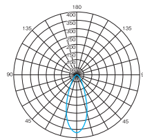
LDR5D-W-E17(昼光色)
