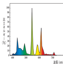
3波長形昼白色 (EX-N) Ra84
