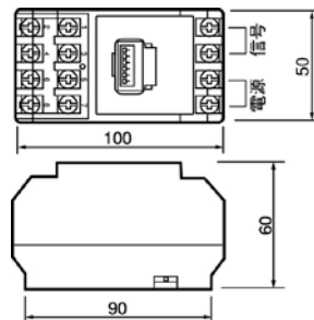
JIS協約寸法(2個用)
