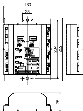
JIS協約寸法(2個用)
