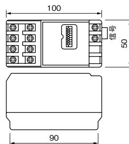
JIS協約寸法(2個用)
