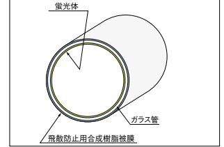
ランプ断面図
