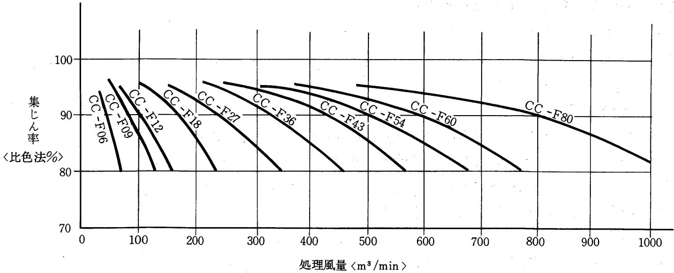
〈集じん率—処理風量特性曲線〉
