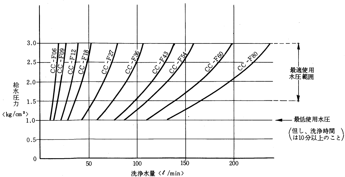
〈洗浄水圧—水量関係曲線〉
