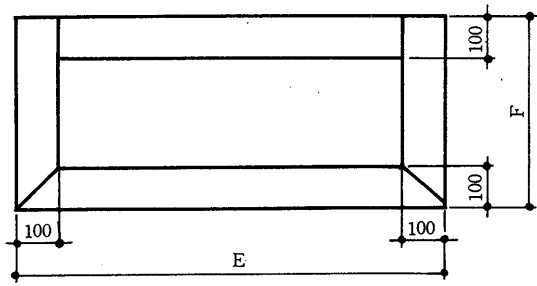
据付台寸法図<参考>
