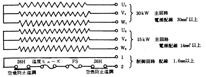
結線図
