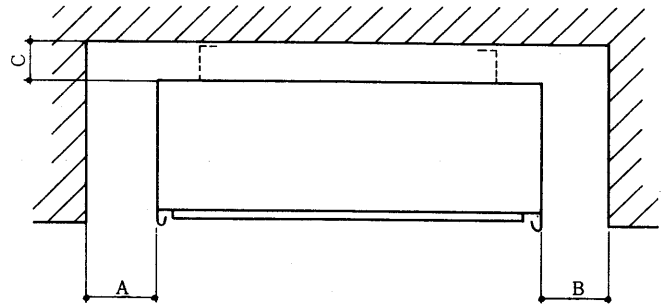
吸込みに必要な最少寸法
