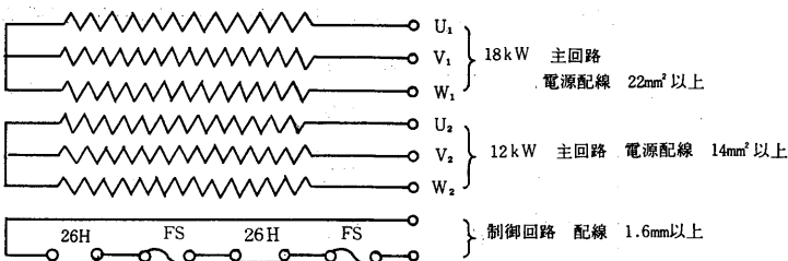
結線図
