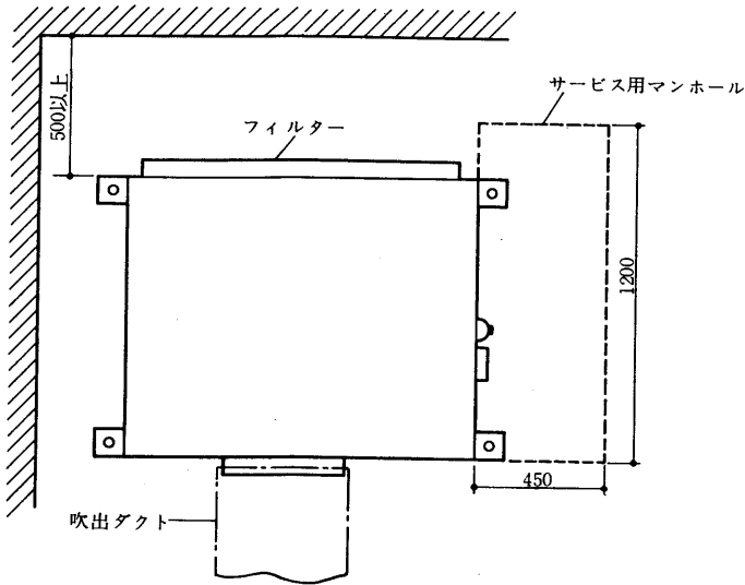
吸込みに必要な最少寸法
