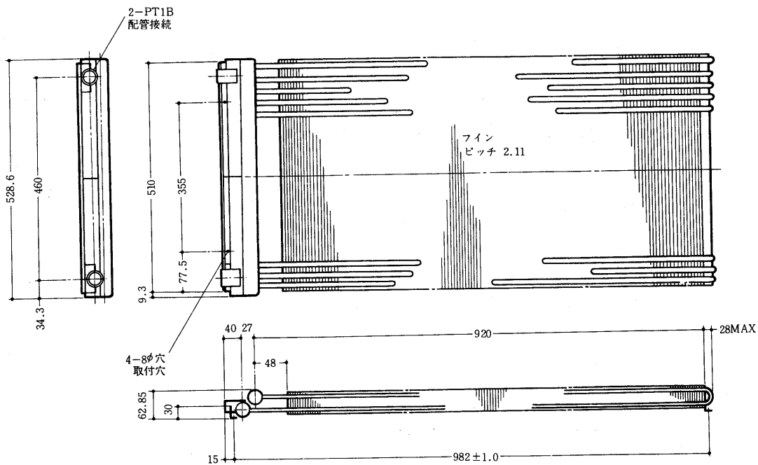
GT-80M・F, GAT-80形<2列>温水・蒸気兼用
