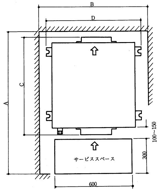
据付けサービスに必要な最小寸法<単位mm>
