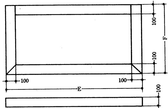
据付台寸法図
