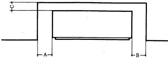
吸込みに必要な最小寸法
