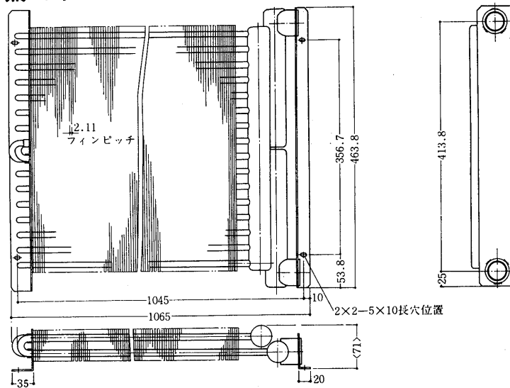
GT-80M・F, GAT-80形<2列>温水・蒸気兼用
