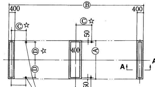
主電動機用コンジット 取り出し位置 〈基礎図〉
