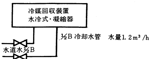
冷媒回収装置水冷式凝縮器水配管系統図
