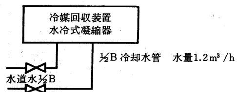
冷媒回収装置水冷式凝縮器水配管系統図
