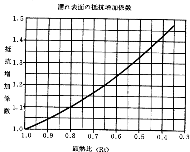
濡れ表面の抵抗増加係数
