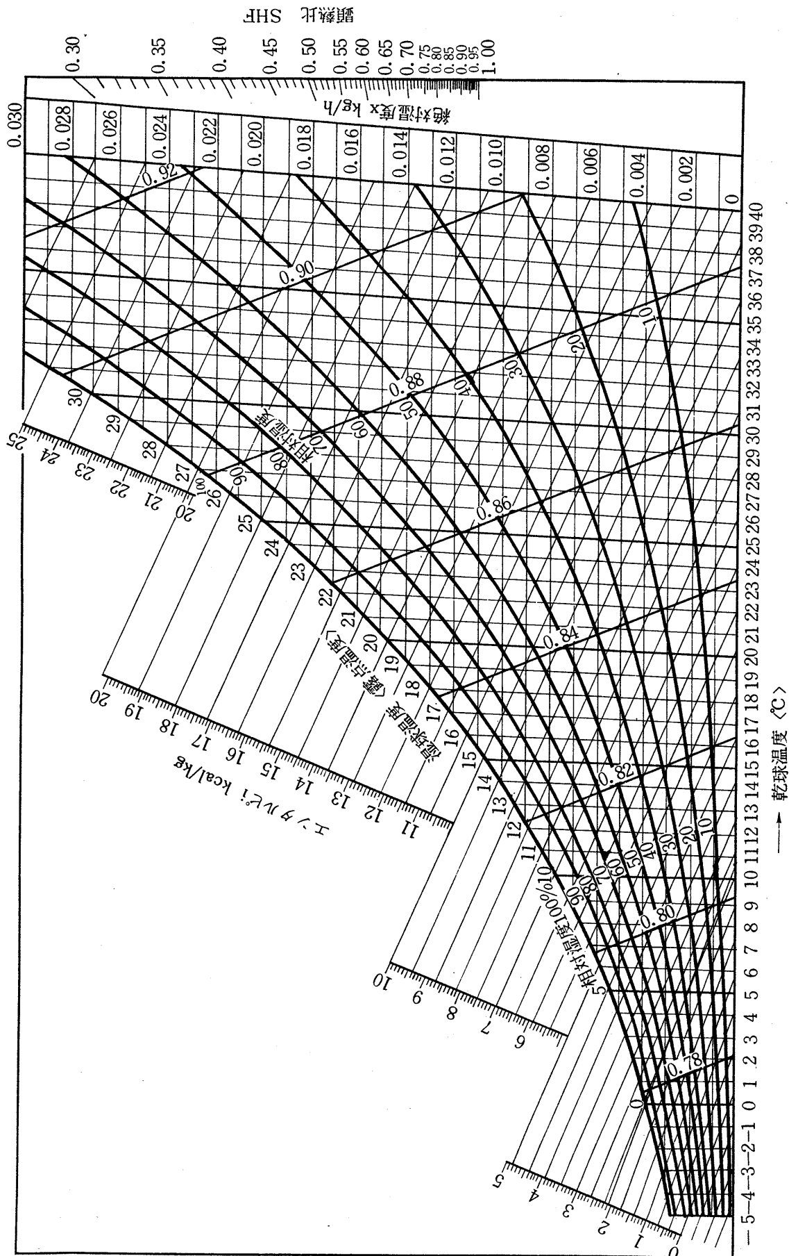
図2 空気線図
