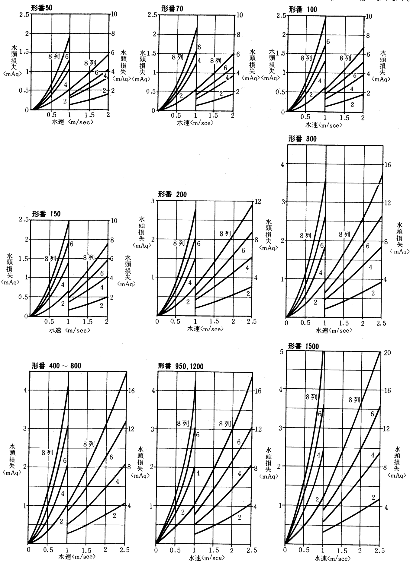
図7 冷温水コイル管内損失水頭
