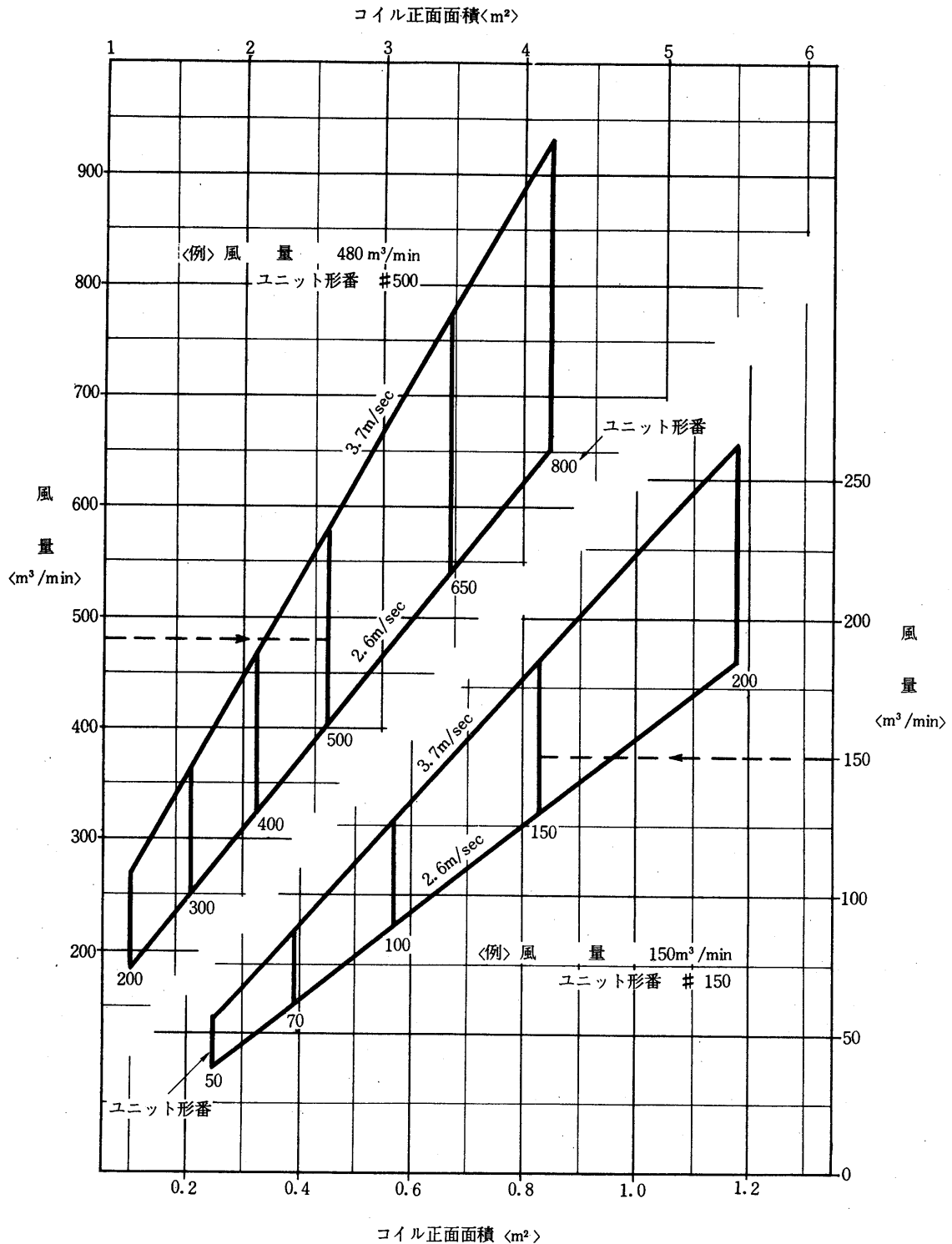
図1 ユニット形番選定図〈形番50～800〉
